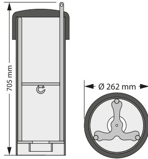
Abmessungen Schutzgehäuse
